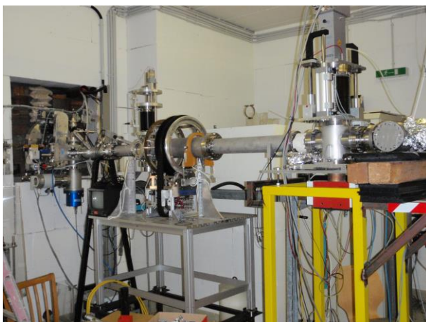
De versnellerbuis
