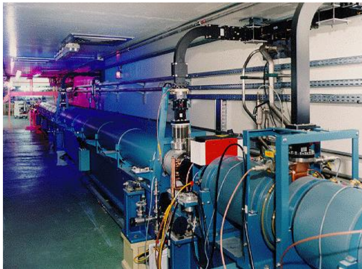
De lineaire versneller (12 m lang) waarmee de elektronen versneld worden voor dat ze het grote synchrotron ingaan.
